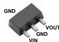
TO-243AA (SOT-89) (N8)
