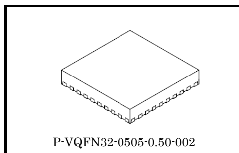
TB6569FTG:質量: 0.07 g (標準)
