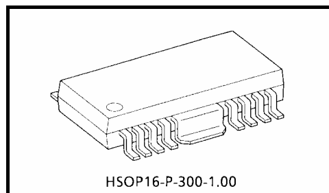
TB6569FG : 質量: 0.5 g (標準)
