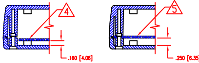
LH57-130 SECTION B-B
