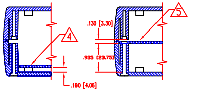
LH57-200 SECTION B-B
