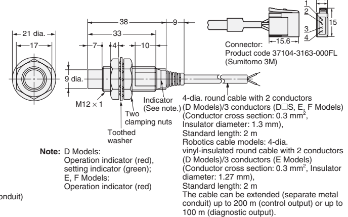
Fig. 9 : E2E-X8MD□ E2E-X5ME□/F□
