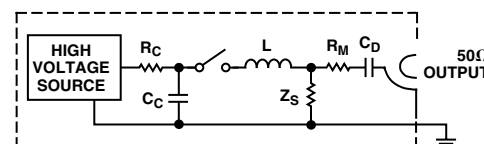
Figure 12. EFT Generator
