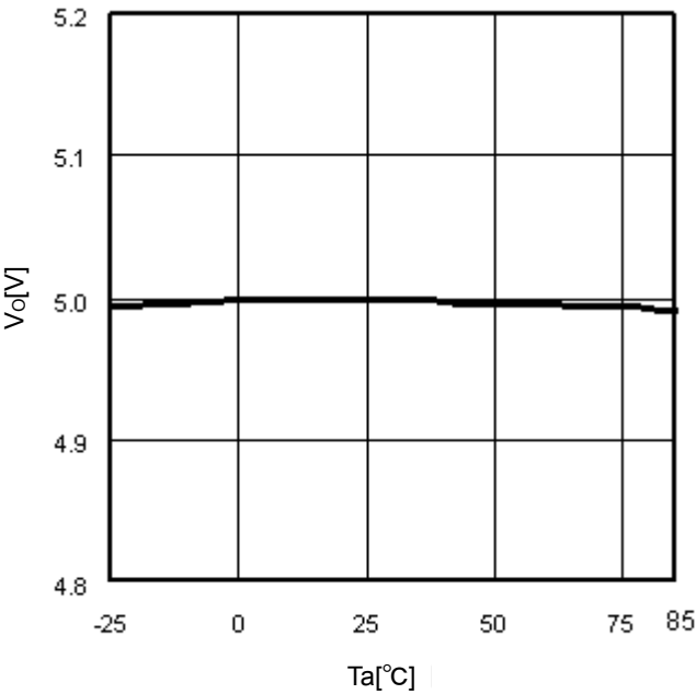
Fig.9 Ta-Vo (Io=0mA)
