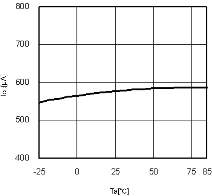
Fig.10 Ta-Icc
