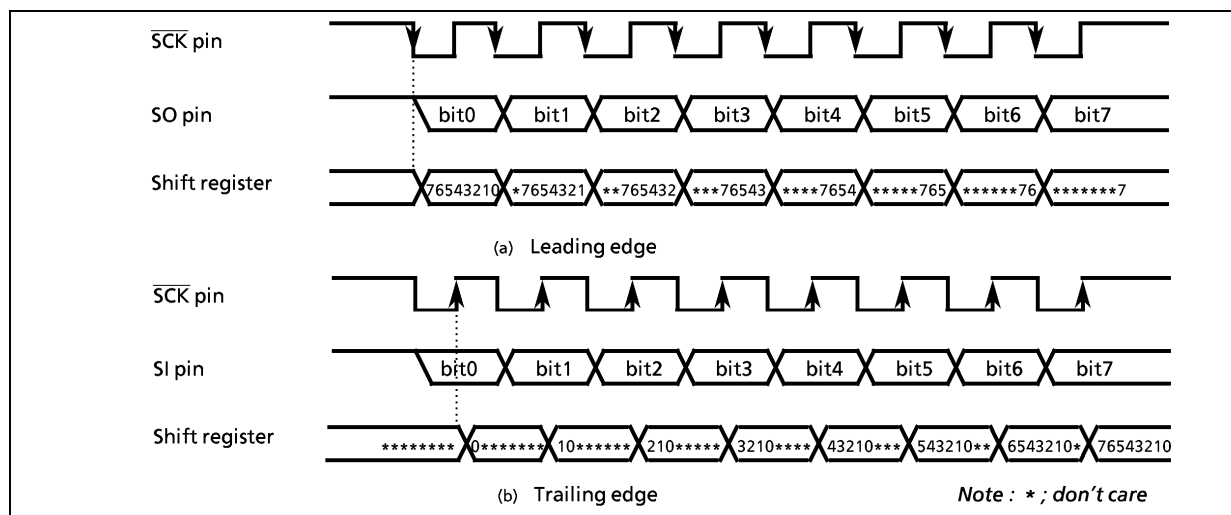
Figure 2-46. Shift edge
