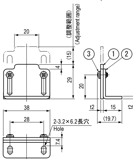
TL-240 スウィングラッチ用受け金具 Receptacle
