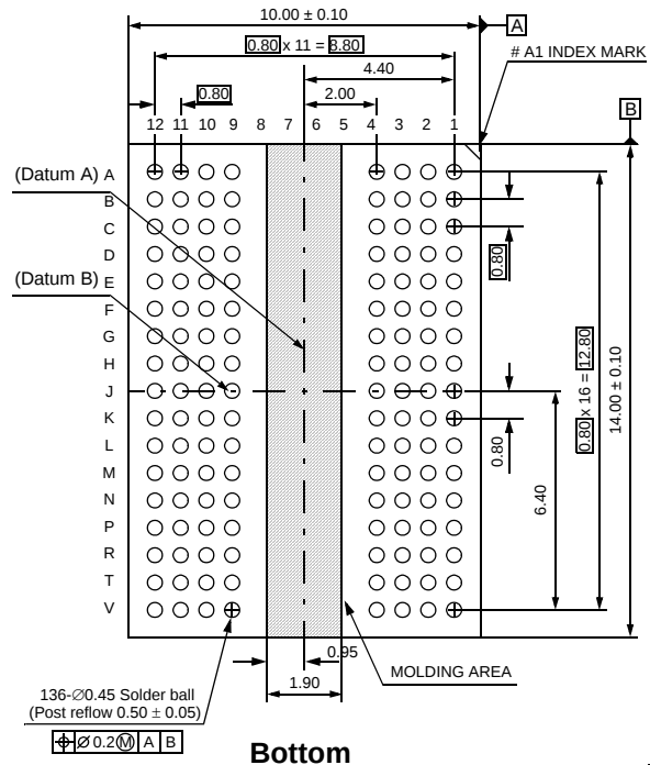
Bottom
