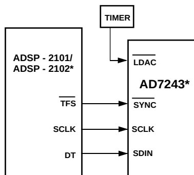
Figure 11. AD7243–ADSP-2101/ADSP-2102
