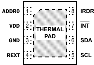
ISL29028A 8 LD ODFN (2.0MMX2.1MMX0.7MM) TOP VIEW
