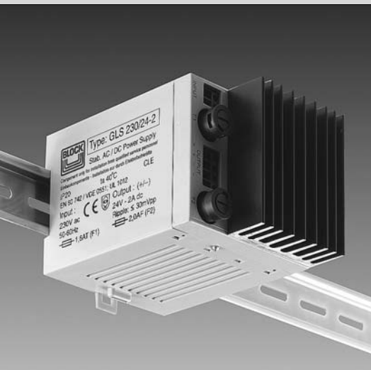
GLS 230/24-2
