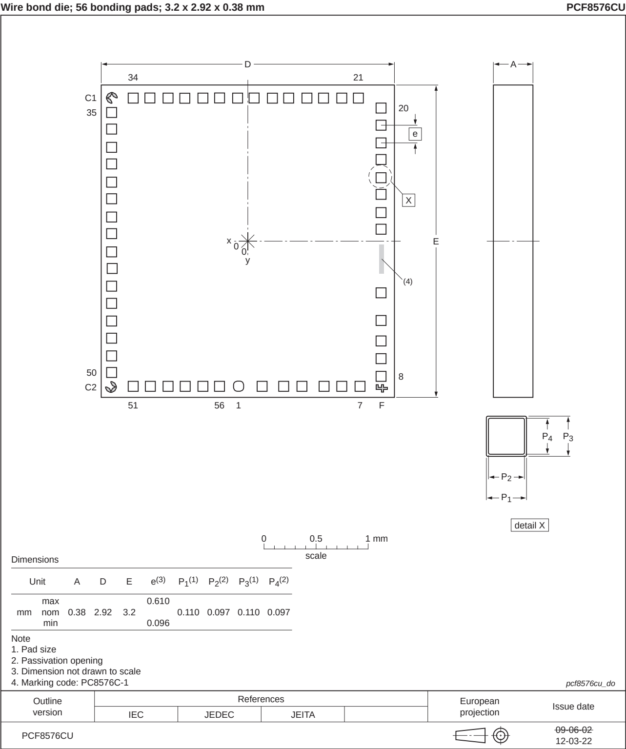
Fig 35. Bare die outline of PCF8576CU/F1
