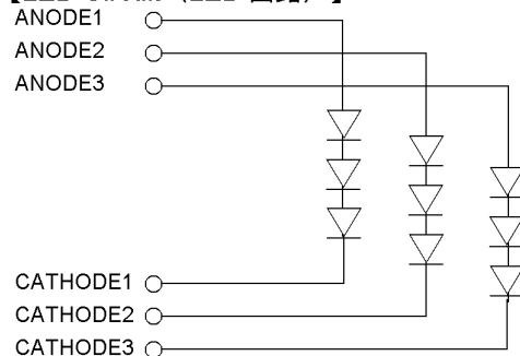
【LED Circuit (LED 回路)】
