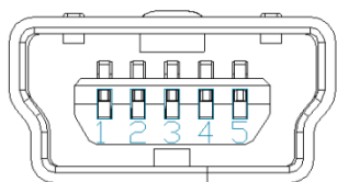
Figure 12: Mini USB Connector
