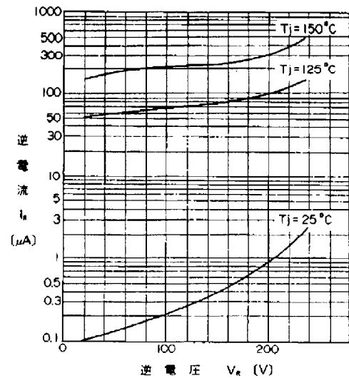
逆特性 (代表特性) Reverse Characteristics
