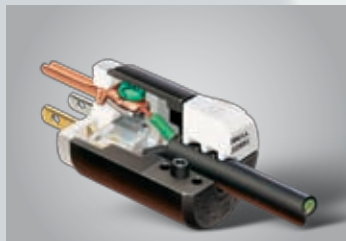
Hubbell Insulgrip®
