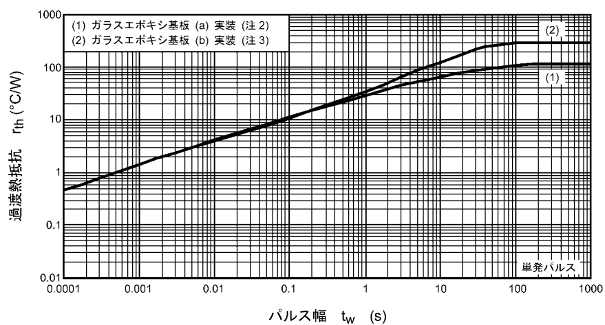
図 8.12 r_{th} - t_w (最大値 (保証値))
