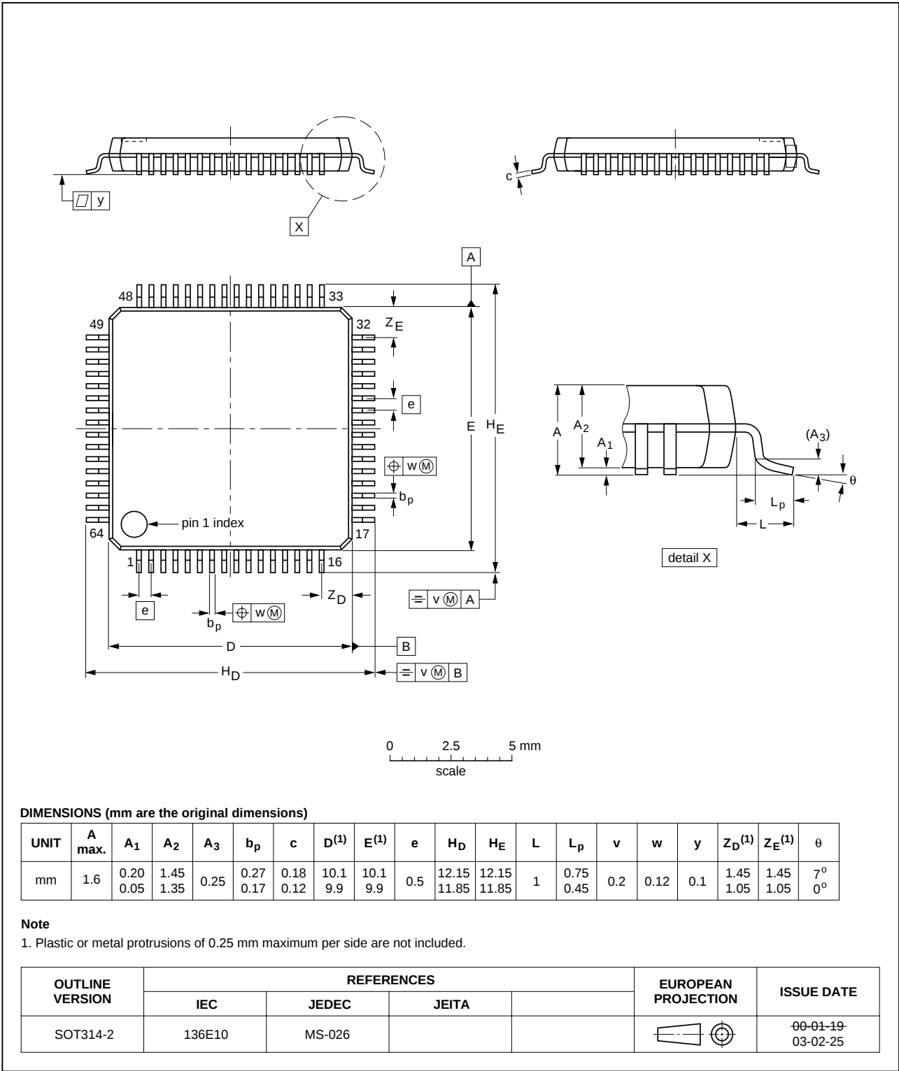
Fig 19. LQFP64 (SOT314-2).
