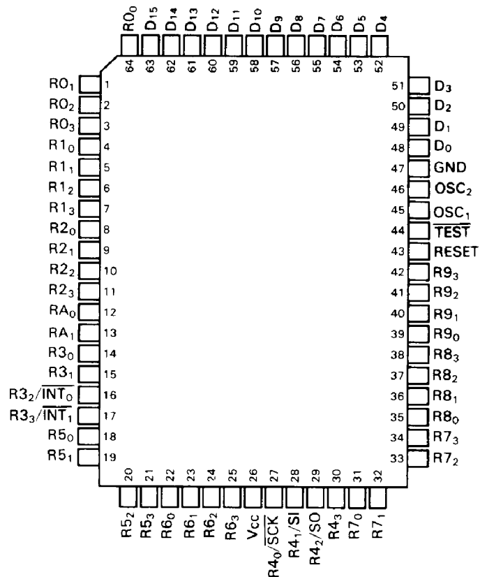
(FP-64)
