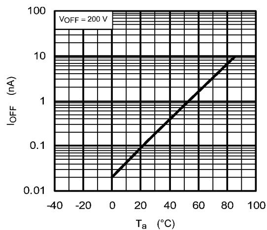
Fig. 14.1.9 I_{OFF} - T_a
