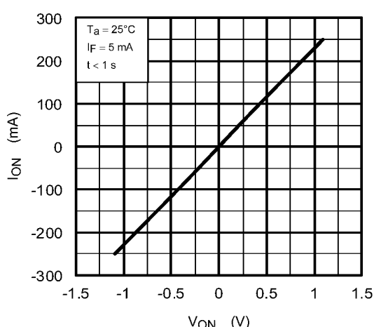
Fig. 14.1.4 I_{ON} - V_{ON}
