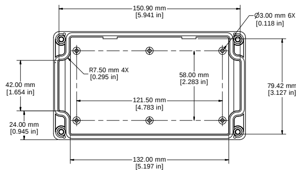
LID - INSIDE
