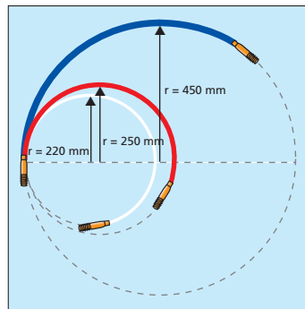
Die Cable Scout+ Biegeradien im Überblick
