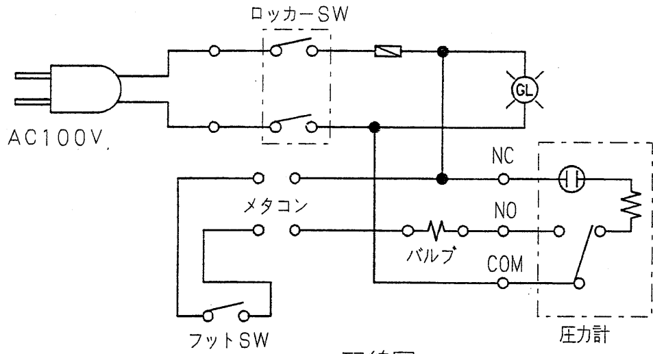
配線図
