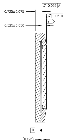
SECTION A-A
