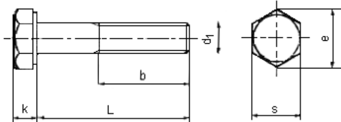
DIN 931/ISO 4014
