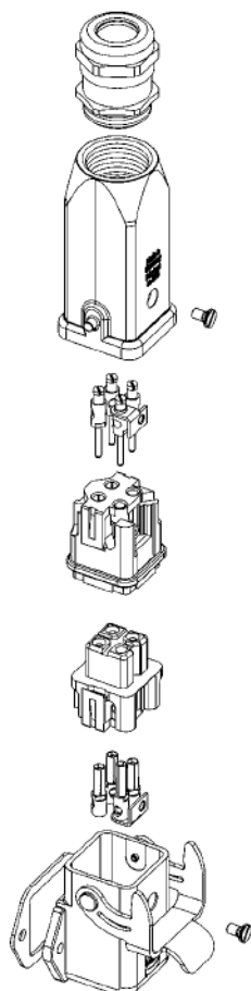
Han® 3 A
