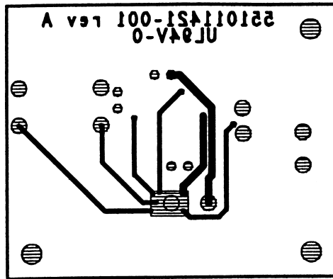
Bottom Layer
