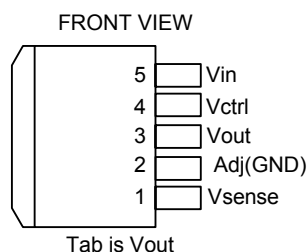
TO263-L
