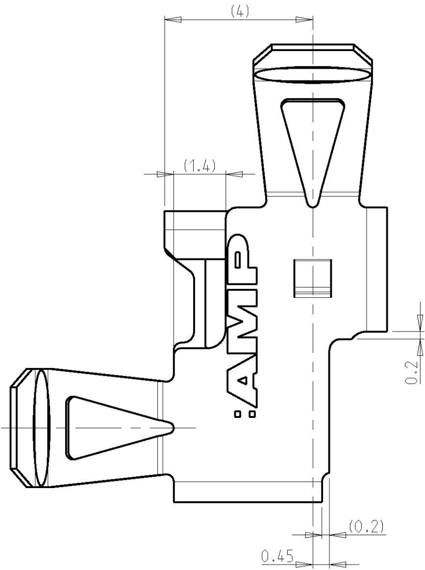
2 RECEPTACLE, CONVERSATION KIT FROM -1 2 BUCHSEN, UMBBAUSATZ VON -1
