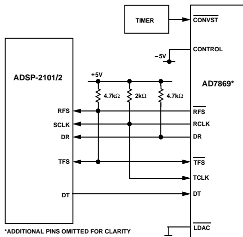
Figure 17. AD7869–ADSP-2101/ADSP-2102 Interface
