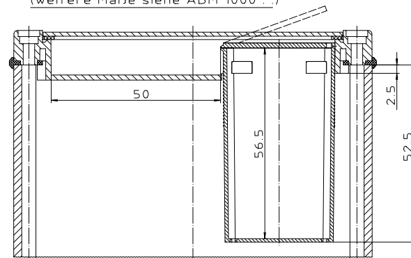
ABM 1000 .. BE (weitere Maße siehe ABM 1000 ..)
