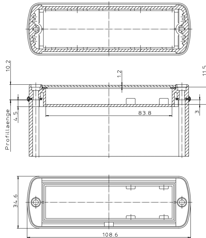
Ansicht ohne Profilkappe bzw. ohne Profilklappe
