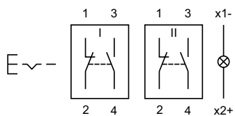
Wiring diagram 24
