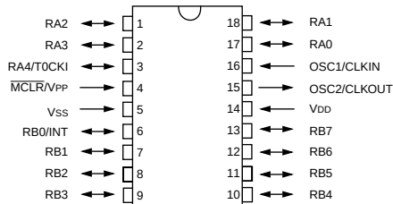
PIC16C61
