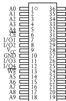
36-pin SOJ (400 mil)
