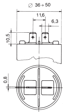
Fig. 2 Faston semplice 6,3 x 0,8 mm
