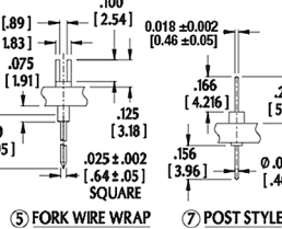
⑤ FORK WIRE WRAP
