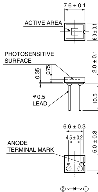
④ S1337-33BR
