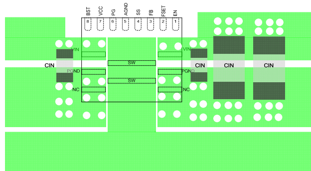
Top Layer
