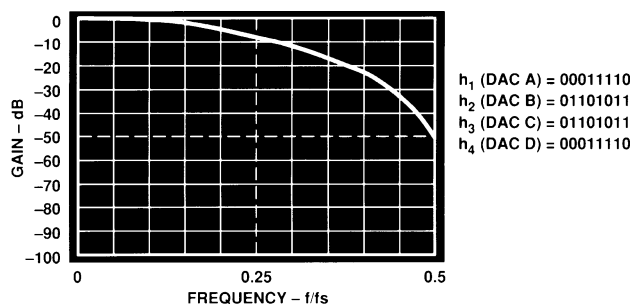
Figure 20. Actual Response
