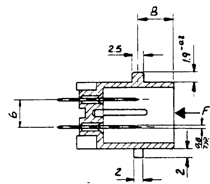
SECCION A-A
