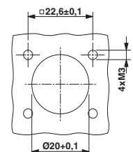
Einbaumaße: RF-1.S..8AAK00 , RF-1.P..8AAK00
