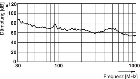
Schirmdämpfungskurve in Anlehnung an DIN EN 50289-1-6 (Kabelstecker und Gerätestecker gewinkelt auf Grundplatte)
