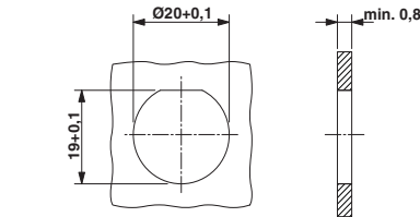
RC-00000006100, Montage Bohrung mit Verdrehenschutz und Kontermutter (Empfehlung bei Einbau in Stahlblechwand)
