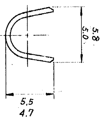
断面 B-B
