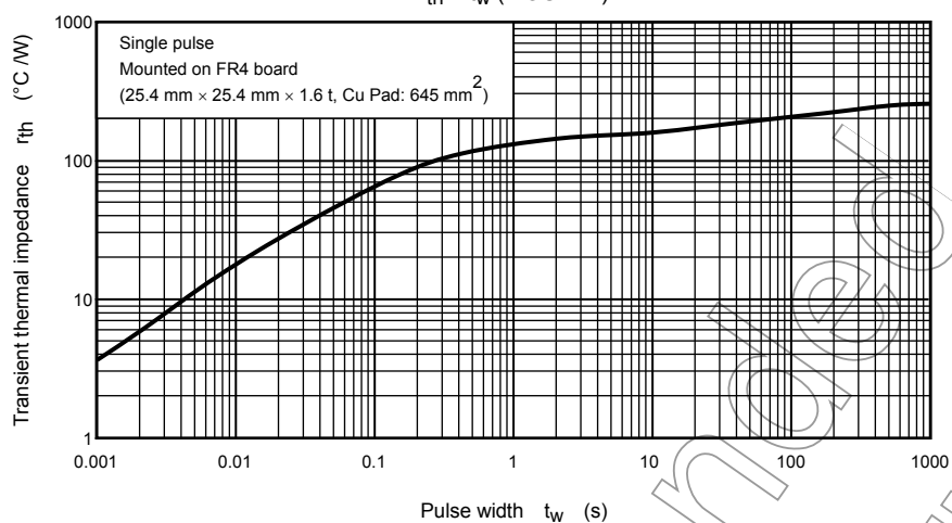
r_{th} - t_w (MOSFET)
