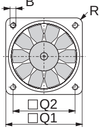
D591T, 601T, 603T, 604T 24 VDC
