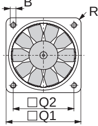
D591Q, 601Q, 603Q, 604Q 12 VDC
