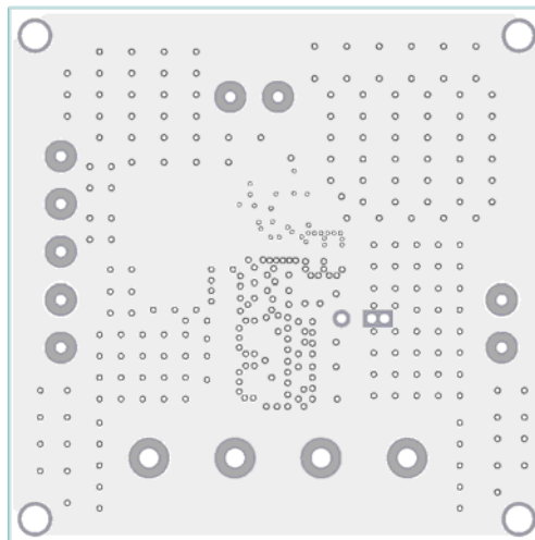
Inner1 Layer
