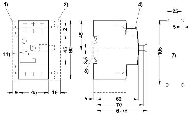
Circuit-breaker J7MN-50
