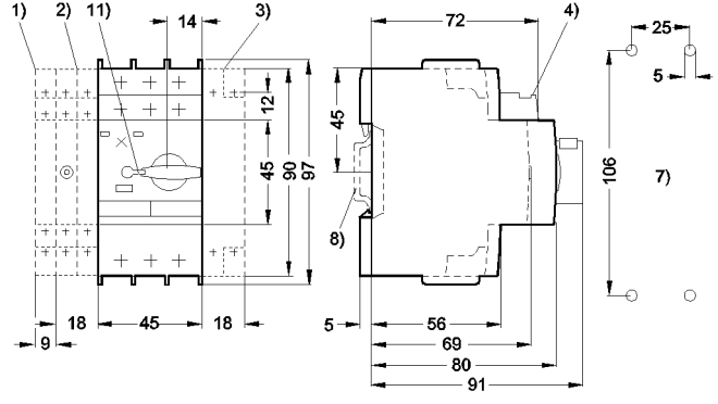
Circuit-breaker J7MN-25
