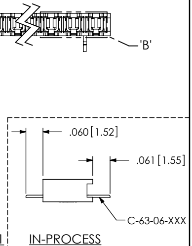
DETAIL 'B' SCALE 12 : 1
