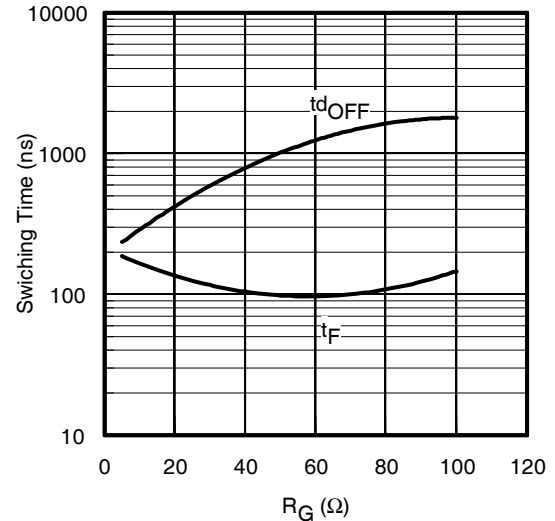
Fig. 16 - Typ. Switching Time vs. R_G T_J = 150^\circ\text{C} ; L = 200\mu\text{H} ; V_{CE} = 600\text{V} ; I_{CE} = 30\text{A} ; V_{GE} = 15\text{V}
