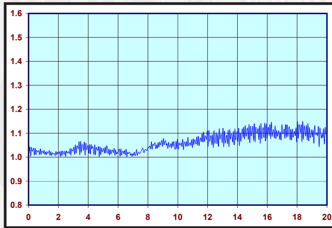
PN: CCSMA-MM-SS402-120 VSWR (S22)
